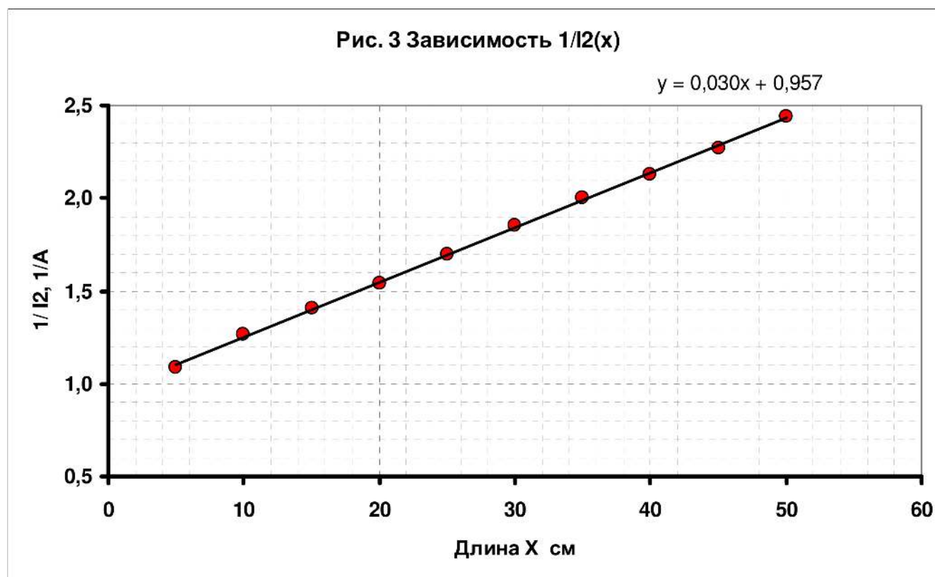
Рис. 3 Зависимость 1/I_2(x)
