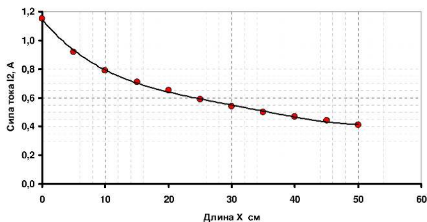
Рис. 2 Зависимость I_2(x)
