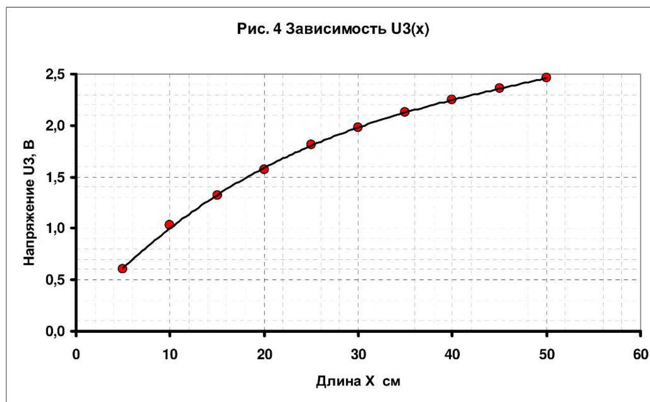
Рис. 4 Зависимость U_3(x)
