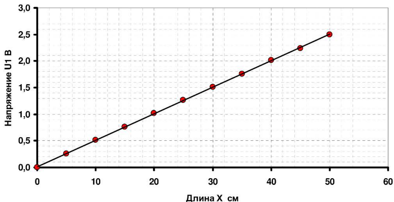
Рис. 1 Зависимость U_1(x)
