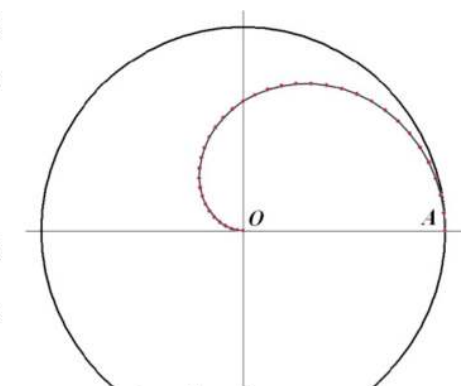
Рис. 7. Общий вид траектории центра масс при горении
