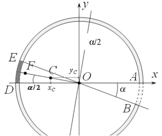
Рис. 2. Вычисление центра масс кольца при горении
