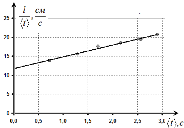
Рис.2 Скатывание цилиндра
