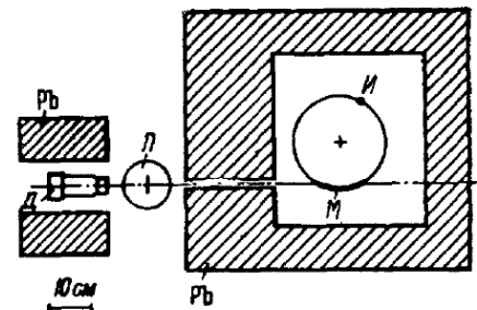
Рис. 2. Геометрия опыта. И — криостат с поглотителем ( T = 88^\circ \text{K} ); М — вращающийся криостат с источником ( T = 88^\circ \text{K} ); Д — детектор; И — источник.
