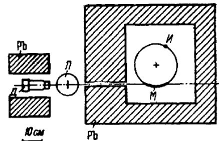
Рис. 2. Геометрия опыта. И — криостат с поглотителем ( T = 88^\circ \text{K} ); М — вращающийся криостат с источником ( T = 88^\circ \text{K} ); Д — детектор; Пб — источник.
