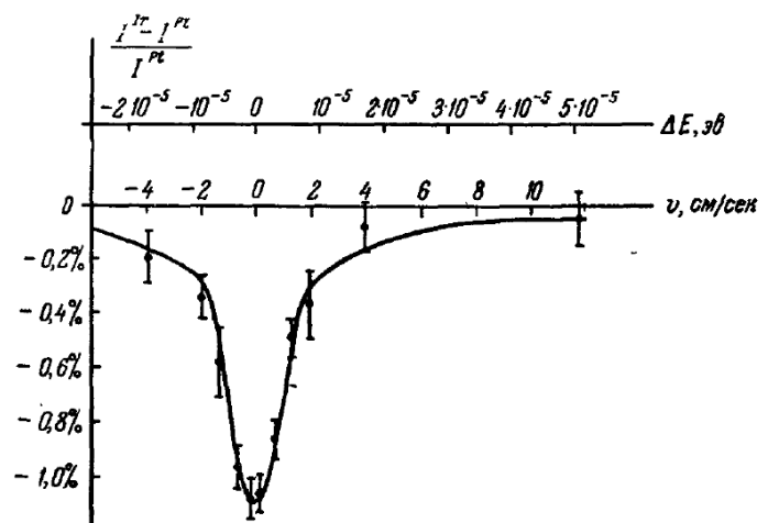
Рис. 3. Относительная разность интенсивностей \gamma -излучения, проходящего через иридиевый и платиновый поглотители, в функции относительной скорости источника и поглотителя.
